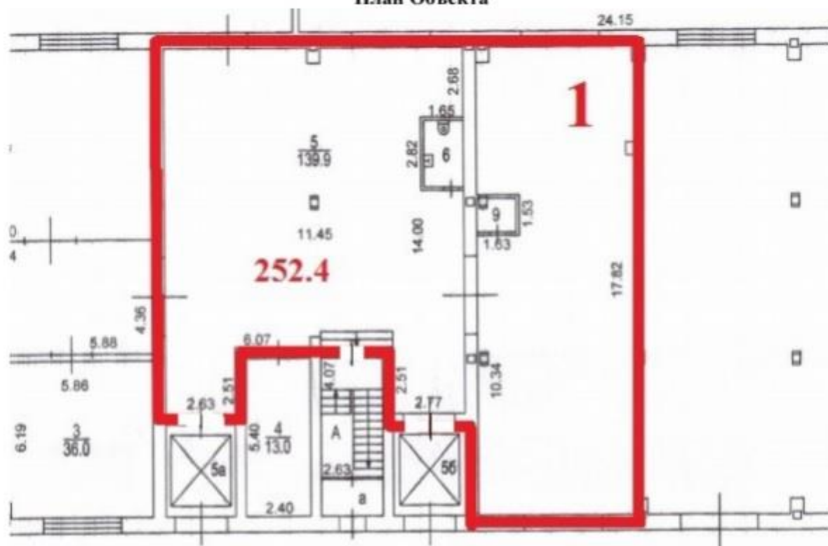
План Объекта
